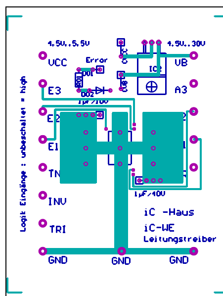
Bild 8: Demo-Board (Lötseite)
