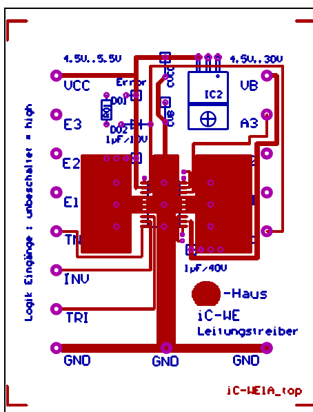
Bild 7: Demo-Board (Bestückungsseite)
